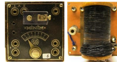
6-Minim-Krystalapparat-nej afstemt
