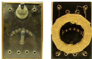
129-Ukendt-Krystalapparat-nej afstemt
