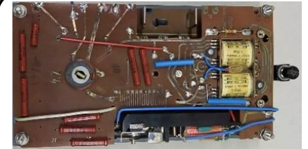
717-Goerz-Unigor 3p 1967
