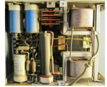
730-Eltra-216-ohmmeter 1950
