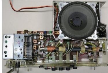
255-Blaupunkt-Derby-670
