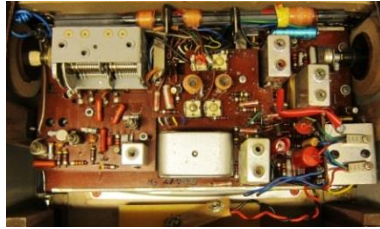
50-AGA-Transistor-2800
