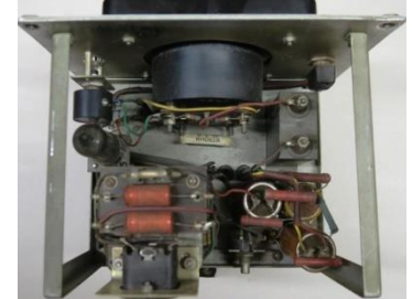
733-Philips-Rørvoltmeter-GM4132 1939
