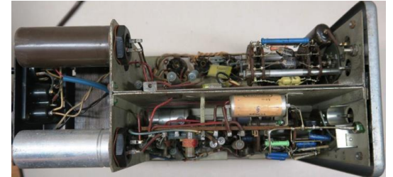
713-Metrix-Oscilloskop-OX722 1990
