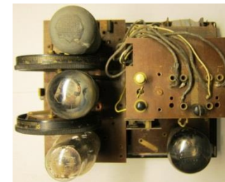
66-Telefunken-Arcolette-3W
