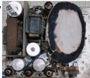
247-Philips-Autoradio-NDK491V
